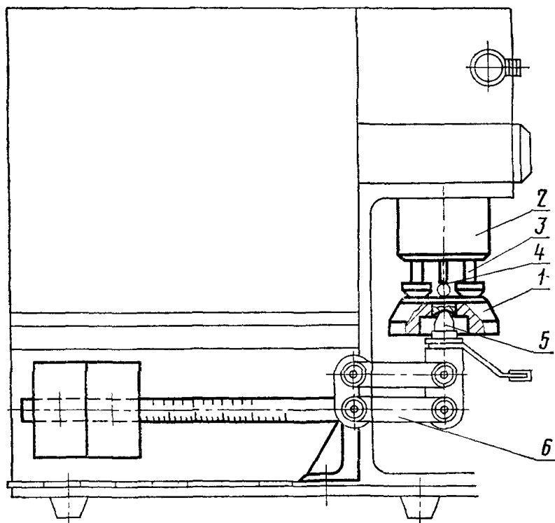
1—палец; 2—истирающая головка; 3—бегунок; 4—устройство для натяжения используемой или абразивной ткани; 5—опора палец; 6—рычажно-грузовая система для создания нормального давления.
