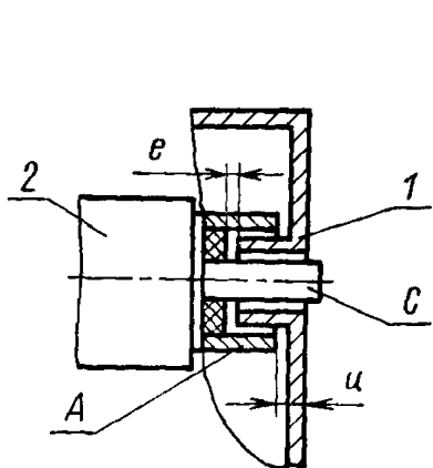
1—цилиндрический экран; 2—испытуемая лампа; А, С—контактные поверхности выводов электродов испытуемой лампы.
