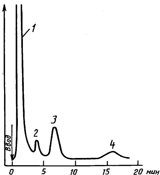
Типовая хроматограмма этиленгликоля с использованием колонки I
