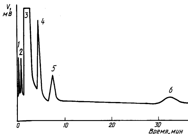
Типовая хроматограмма этиленгликоля с использованием колонки II
