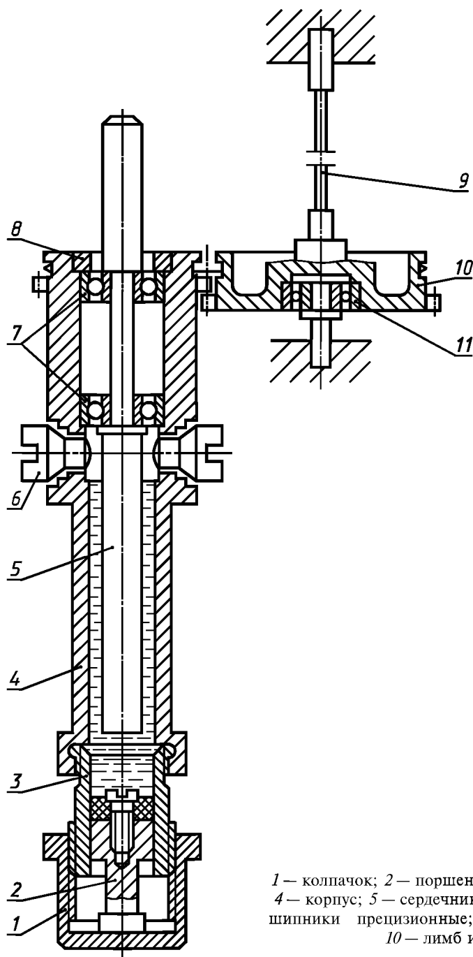
Схема ротационного вискозиметра ПВР-1
