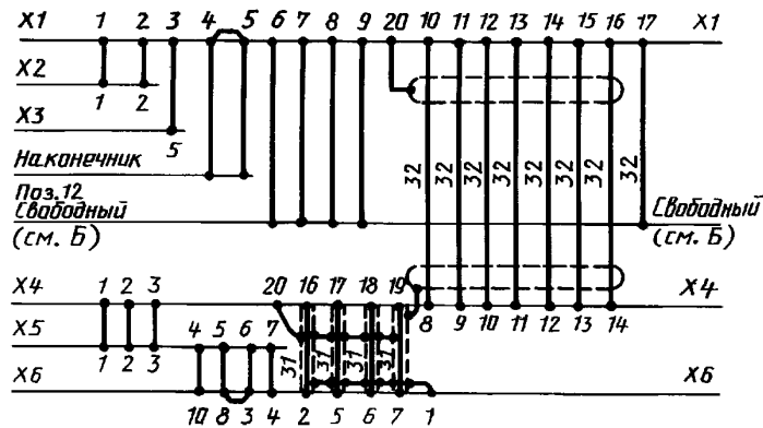
Провод поз. 30, кроме указанных особо.
