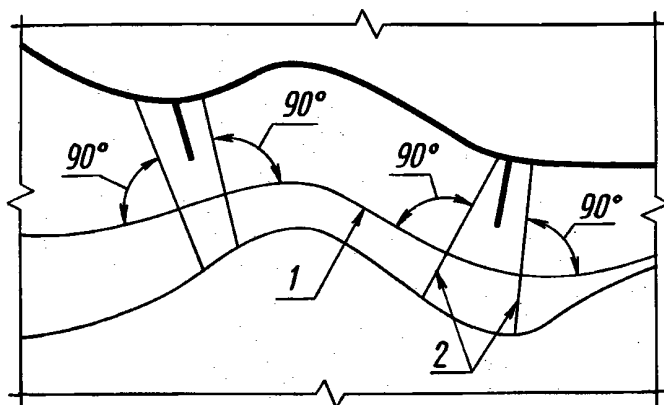
1 — горизонталь; 2 — линия наибольшего ската.
