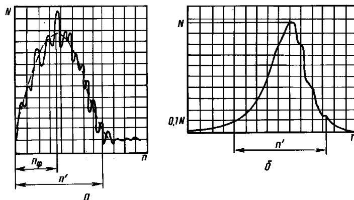
a — с крутым фронтом; б — с пологим фронтом
