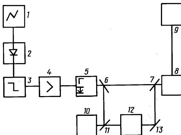
1 — осциллограф; 2 — частотный детектор; 3 — ограничитель; 4 — полосовой усилитель на частоту 30 мГц; полоса пропускания 0,5 мГц; 5 — фотоприемник; 6, 7, 11 — зеркала с коэффициентом отражения не менее 50 %; 8 — фокусирующая система; 9 — испытуемое изделие; 10 — газоприемник; 12 — устройство для сдвига частоты; 13 — зеркало с коэффициентом отражения не менее 90 %
