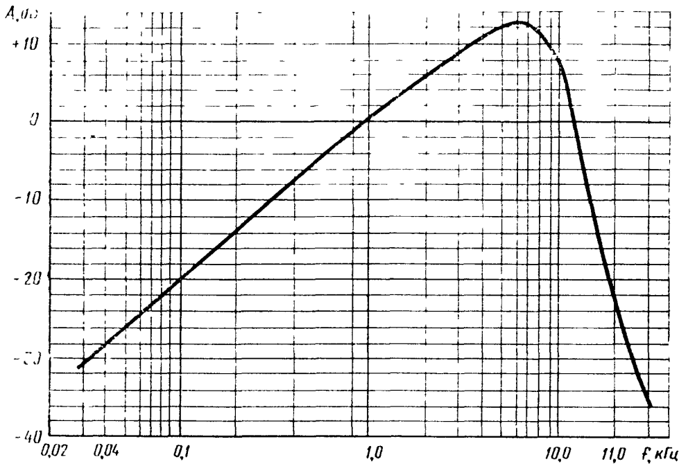
Амплитудно-частотная характеристика психометрического фильтра
