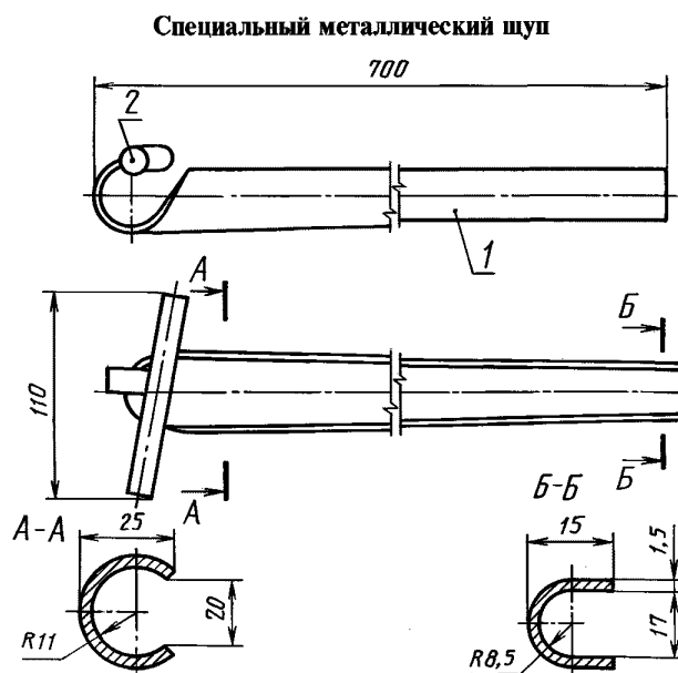
1 — лоток, 2 — ручка
