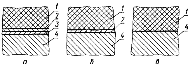
а — при применении двух клеев (методы А и В); б — при применении одного клея; в — при бесклеевом крепении (методы А и В), 1 — резина; 2 — клей, 3 — праймер; 4 — металл
