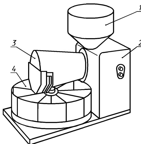
Делитель типа ДСМ-1
