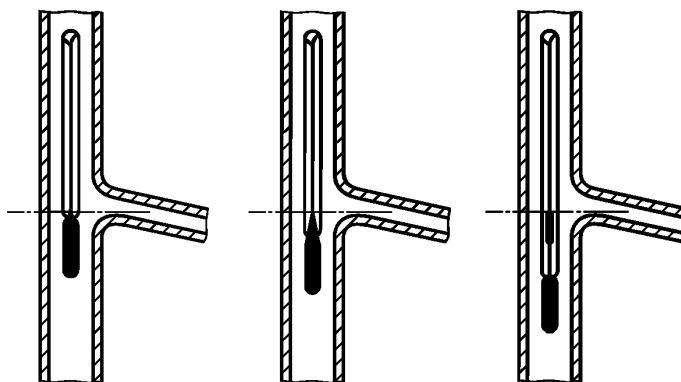
Рисунок 5 — Положение термометра в перегонной колбе
