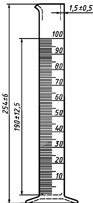
Рисунок 4 — Мерный цилиндр вместимостью 100 см 3 , с ценой деления 1 см 3 , допуск ±1,0 см 3
