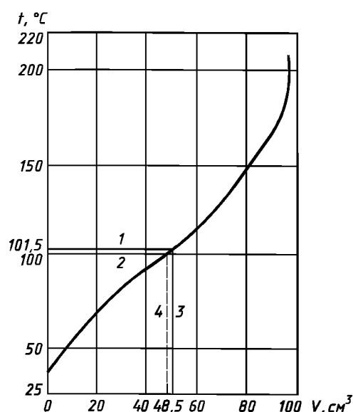
Рисунок Б.1 — Кривая перегонки
