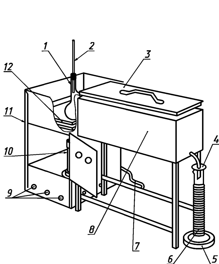
1 — колба для перегонки; 2 — термометр; 3 — крышка бани; 4 — фильтровальная бумага; 5 — подставка; 6 — мерный цилиндр; 7 — газопровод; 8 — охлаждающая баня; 9 — вентиляционные отверстия; 10 — горелка; 11 — кожух; 12 — асбестовая прокладка
