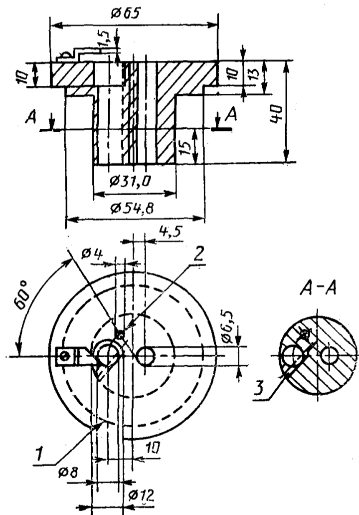
1 — щель, позволяющая отсчитывать температуру вплоть до минус 30°C; 2 — соединение с атмосферой; 3 — зажим из нержавеющей стали для закрепления термометра
