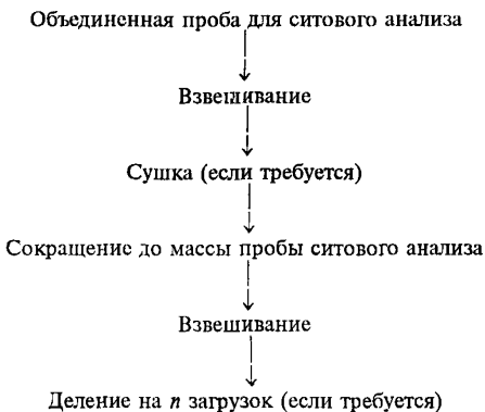
Рисунок 1 — Схема подготовки объединенной пробы к ситовому анализу
