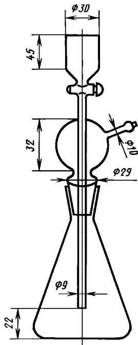
Прибор для растворения металлического олова
