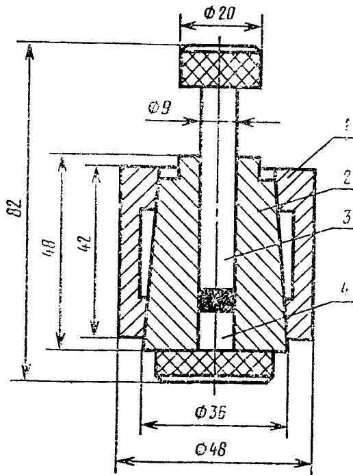
1—сбойма; 2—вставка-матрица; 3—верхний пуансон; 4—нижний пуансон
