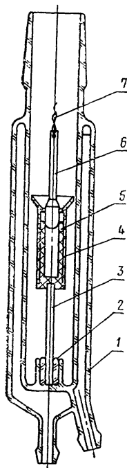
1 — кварцевая водородохлаждаемая колба; 2 — кварцевая вставка (см. черт. 13); 3 — графитовый держатель; 4 — графитовый экран; 5 — графитовый тигель; 6 — графитовая крышка; 7 — молибденовая проволока диаметром 0,8—1 мм
