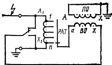
РАТ — регулировочный автотрансформатор
