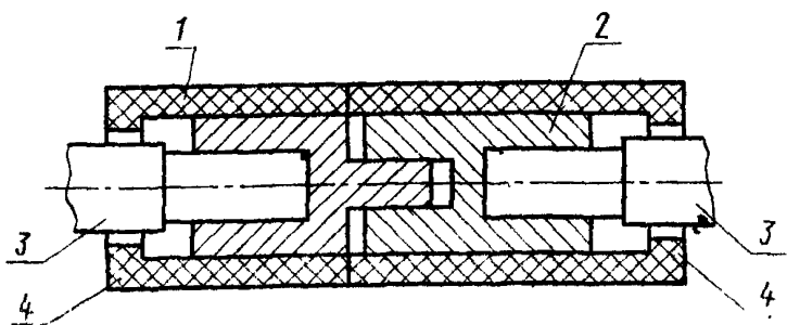
1—вставка; 2—гнездо; 3—кабель; 4—корпус
