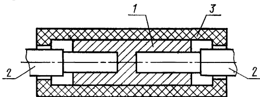
1—сердцевина; 2—кабель; 3—корпус
