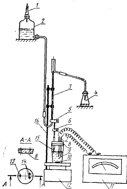
Общий вид потенциметрической установки
