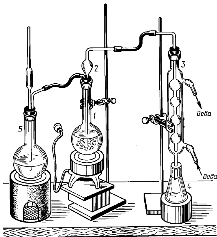
Прибор для отгонки летучих жирных кислот
