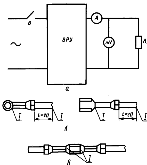
Схема измерения падения напряжения
