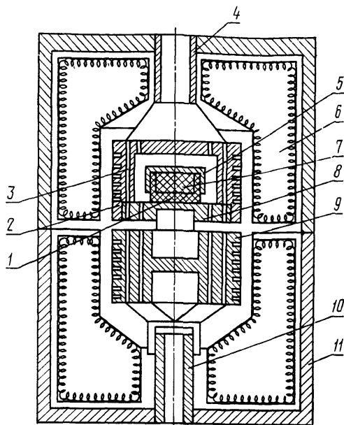
1 — термометр с ампулой; 2 — адиабатная оболочка; 3 — термометр (4 шт.); 4 — входной патрубок; 5 — крышка; 6 — теплозащитная оболочка; 7 — образец; 8 — основание; 9 — нагревательный блок; 10 — выходной патрубок; 11 — корпус
