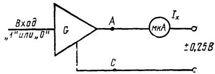
I_x —ток утечки
