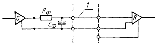
Пример метода формирования сигнала
