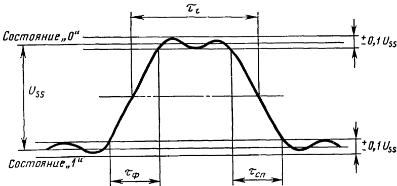
Выходной сигнал генератора для симметричной цепи стыка
