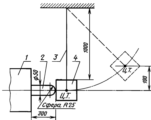
Схема испытания радиационной головки гамма-дефектоскопа на ударную прочность при горизонтальных ударах
