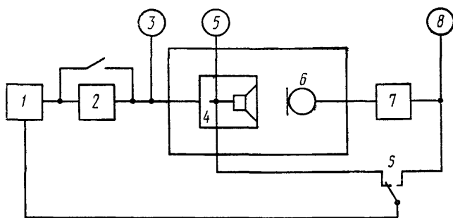
1 — ГНИ с регистрирующим устройством; 2 — усилитель У1; 3, 5, 8 — электронный вольтметр; 4 — измеряемый трехпрограммный приемник; 6 — измерительный микрофон; 7 — усилитель УМ; 9 — переключатель
