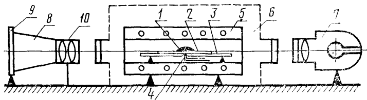
Схема установки для проведения испытаний
