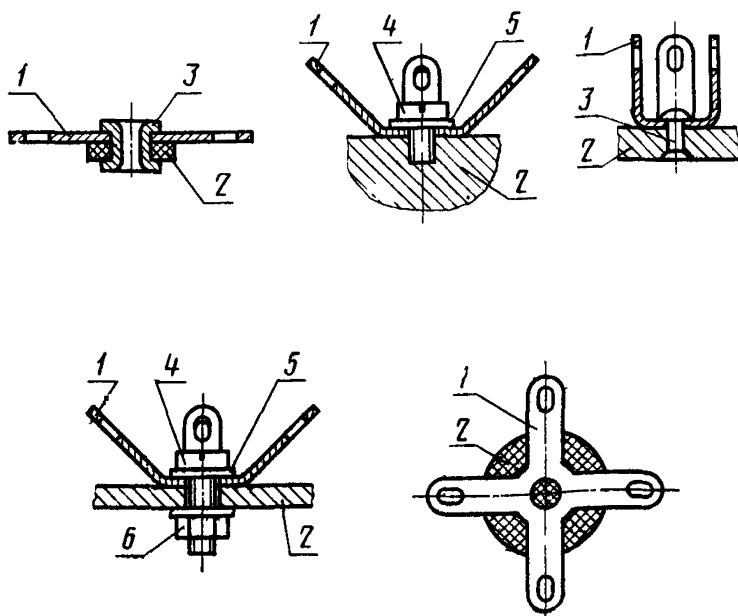
1—лепесток; 2—основание; 3—заклепка; 4—винт; 5—шайба; 6—райка.
