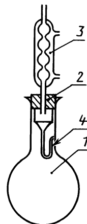
1 — колба; 2 — резиновая пробка; 3 — холодильник; 4 — градуированный приемник
