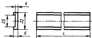
Размеры в мм
