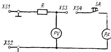
РА—амперметр; PV—вольтметр.
