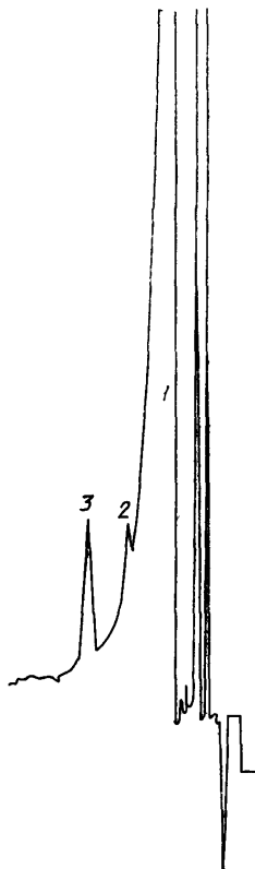
1—пропилен; 2—изобутан; 3— n -бутан
