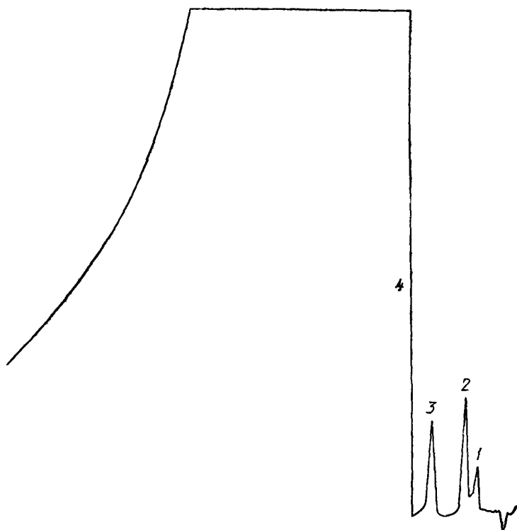
1—окись углерода; 2—метан; 3—двуокись углерода; 4—этилен
