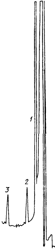
1—этилен, 2—пропадиен, 3—бутадиен-1,3
