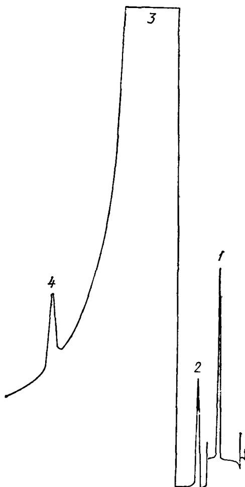
1—метан; 2—этан; 3—этилен; 4—пропилен
