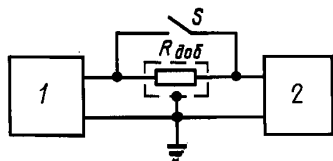
Схема определения входного сопротивления
