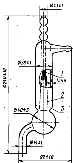
Насос водоструйный
