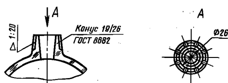
Варианты исполнения крышки
