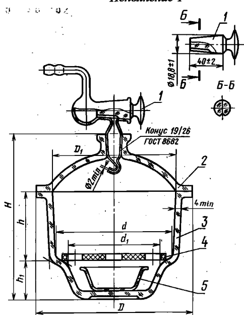
Варианты исполнения крышки
