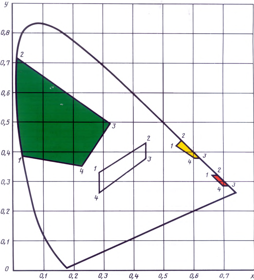
Черт. 1
