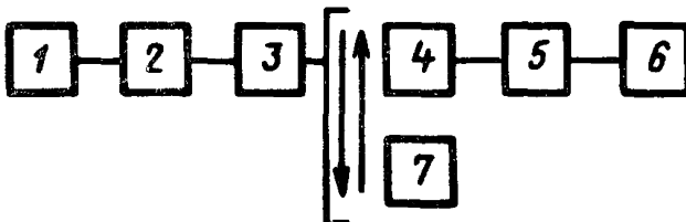
1 — светоизмерительная лампа с системой питания и контроля тока 2 — модулятор 3 — монохроматор 4 — первичный измерительный преобразователь исследуемого средства измерения 5 — селективный усилитель 6 — система регистрации 7 — контрольное средство измерений
