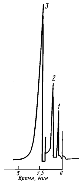
Типовая хроматограмма ацетона при определении массовой доли воды
