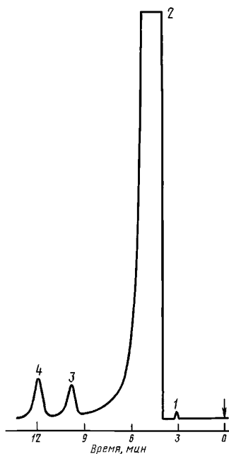
Типовая хроматограмма ацетона
