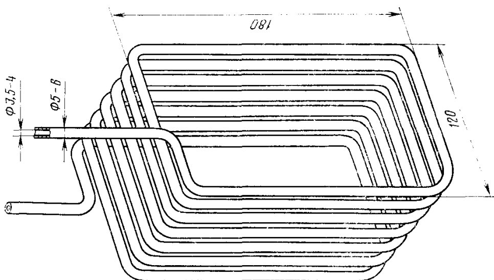
Хроматографическая колонка (молибденовое стекло)
