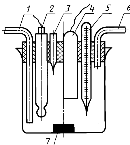
1 — вход раствора; 2 — электрод стеклянный; 3 — микробюретка; 4 — электрод сравнения; 5 — термометр; 6 — выход раствора; 7 — мешалка
