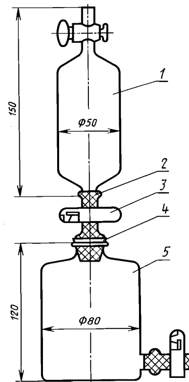
1 — склянка; 2 — шланг; 3 — зажим; 4 — пробка; 5 — склянка с тубусом
