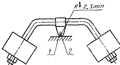
1 — сфера; 2 — образец
