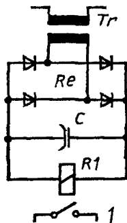
I — выключатель питания ( S на черт. 2а), Re — мост выпрямитель, Tr — трансформатор (обмотка 300/900 витков), R1 — реле (2500 Ом 11000 витков), C — конденсатор (200 мкФ)
