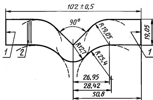
Матрица для испытания прочности на разрыв по п. 21.12
