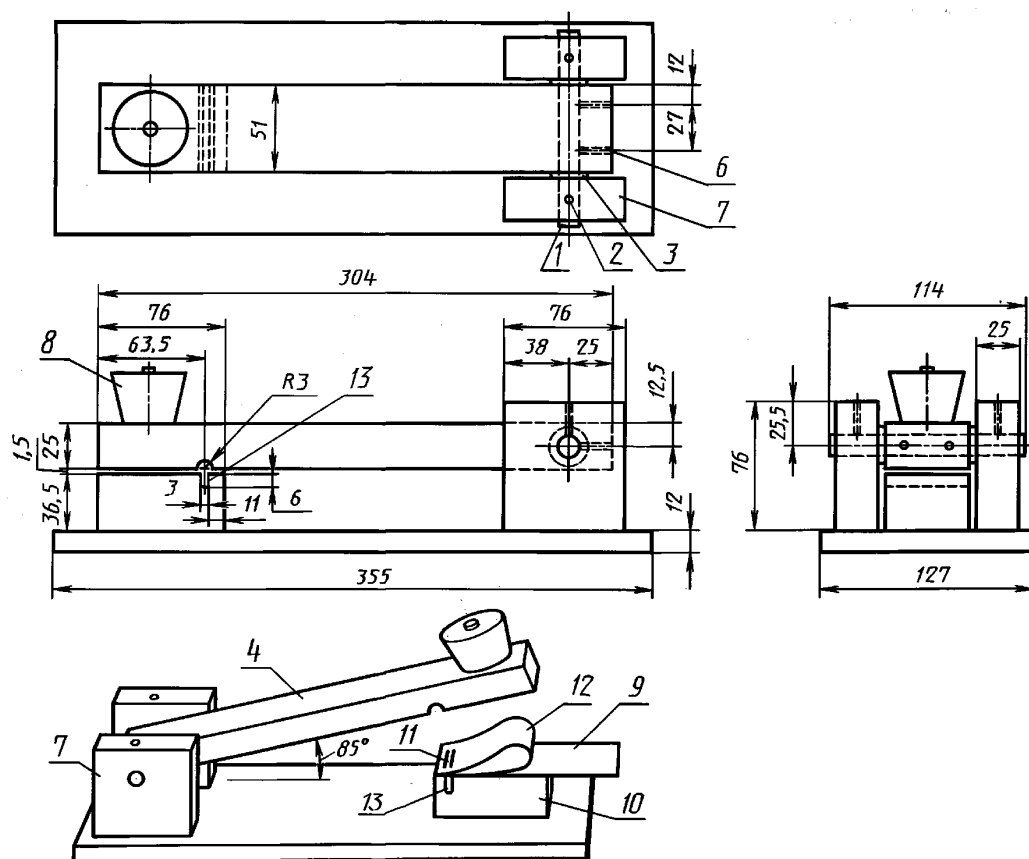
Устройство для испытаний на удар оболочек водонепроницаемых подушек по п. 21.10
