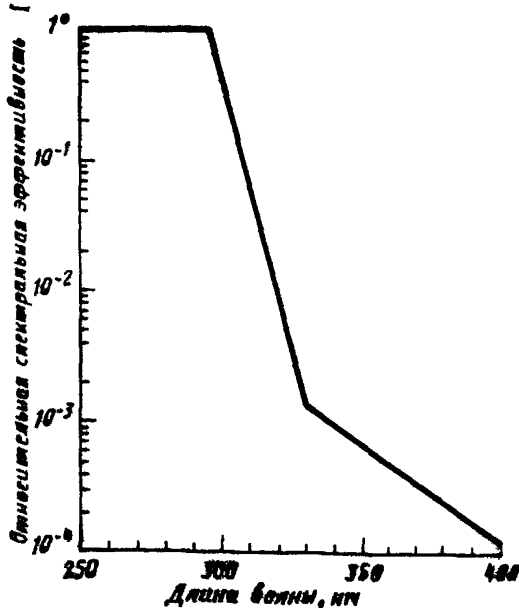
Некоторые значения кривой УФ-воздействия
