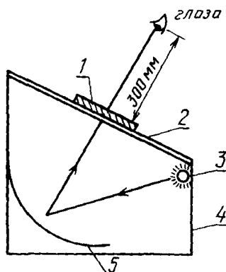
Схема приспособления для освещения пластинок
