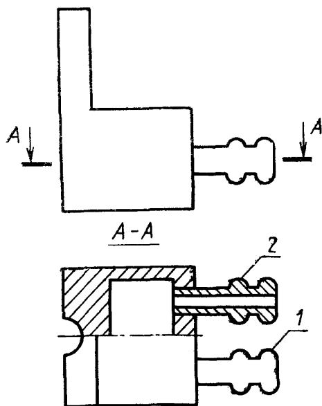
Электрододержатели
