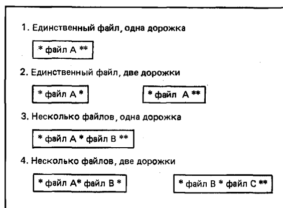
Структура файлов
