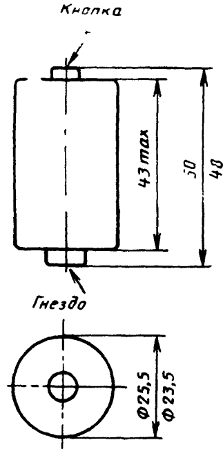
Черт. 64 Контакты-гнездо-стандартная кнопка.
