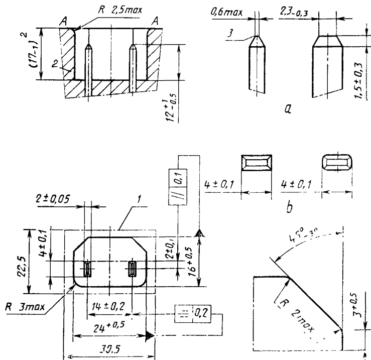
a — концы штырей; b — варианты формы штырей
