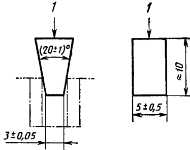
1 — усилие Черт. 9
