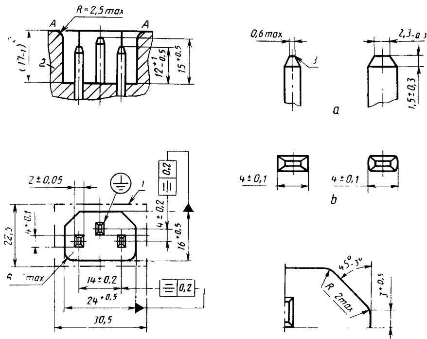
a — вариант исполнения конца штырей; b — варианты формы штырей
