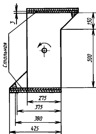
Вращающийся барабан (со стальной плитой толщиной 3 мм)
