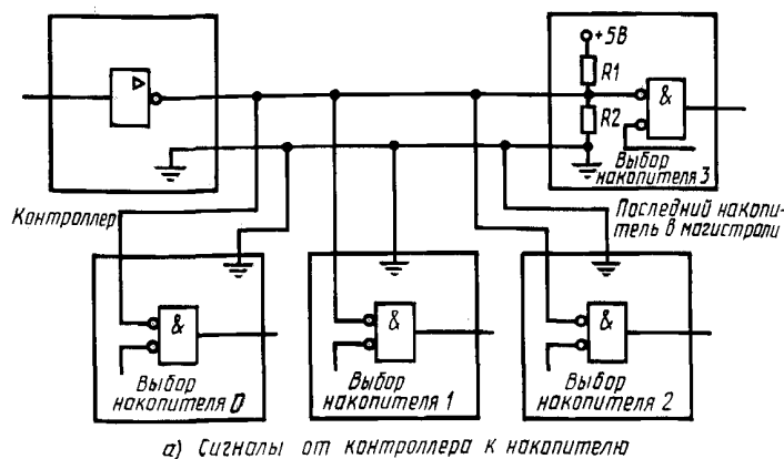
Схема интерфейсных межсоединений
