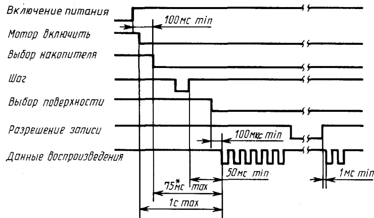
Временная диаграмма начала операции воспроизведения
