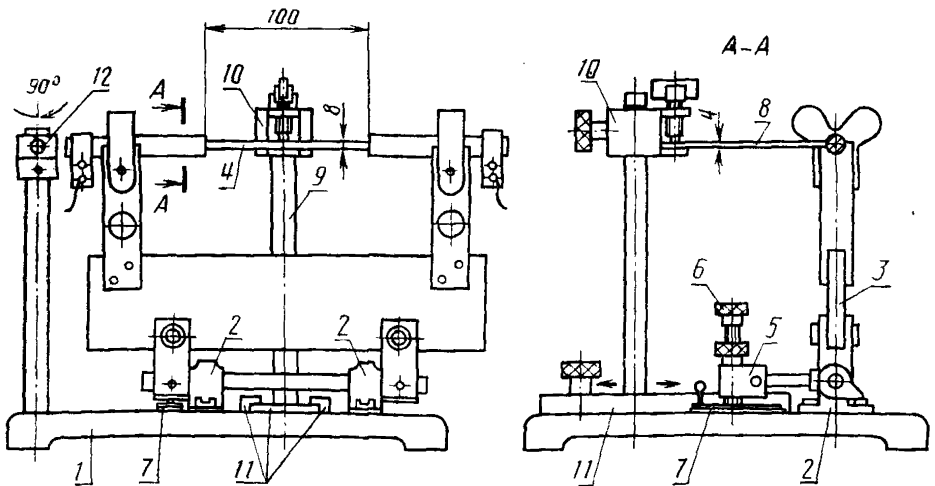
1—опорная плита; 2—подшипники; 3—держатель; 4—накалываемый стержень; 5—противоповзе; 6—опорный винт; 7—поворотная пластина; 8—испытуемый образец; 9—держатель образца; 10—зажим; 11—подвижное основание; 12—поворотный металлический стержень
